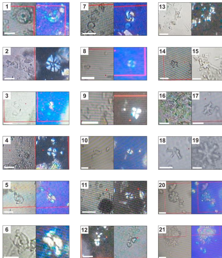
Gambar 5. Foto nannofosil gampingan berumur Neogen-Kuarter di Pulau Timor. (1) Calcidiscus leptoporus ; (2) Hayaster sp.; (3) Umbilicosphaera rotula ; (4) Coccolithus pelagicus ; (5) H. kamptneri ; (6) H. princei ; (7) Dy. productus ; (8) Gy. ericsonii ; (9) Gy. oceanica ; (10) R. producta ; (11) R. pseudoumbilicus ; (12) S. abies ; (13) S. neobies ; (14) D. berggrenii ; (15) D. neorectus ; (16) D. broweri ; (17) D. challengerii ; (18) D. quinquerramus ; (19) D. variabilis ; (20) D. deflandrei ; (21) D. neohamatus . Skala batang 5 µm.
