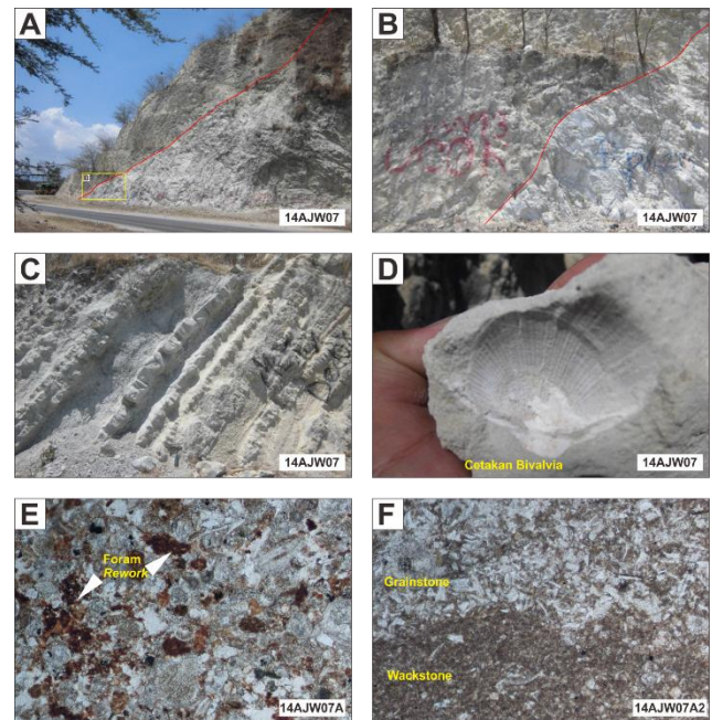
Gambar 2. Foto singkapan Formasi Ofu di daerah Camplong, (A) Singkapan Formasi Ofu di tepi Sungai Mina, (B) Kontak erosional pada batugamping chalky , (C) Perlapisan grainstone foraminifera dan napal (D) Cetakan bivalvia pada grainstone . Sayatan tipis batuan Formasi Ofu (E) Grainstone foraminifera planktonik, dan (F) Kontak antara wackestone dengan grainstone .
