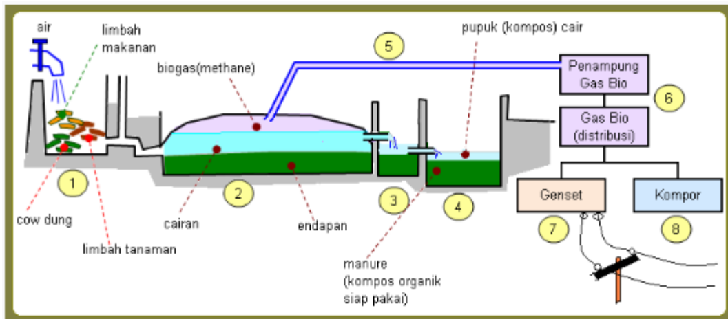
Gambar 1. Proses Pengolahan Biogas
